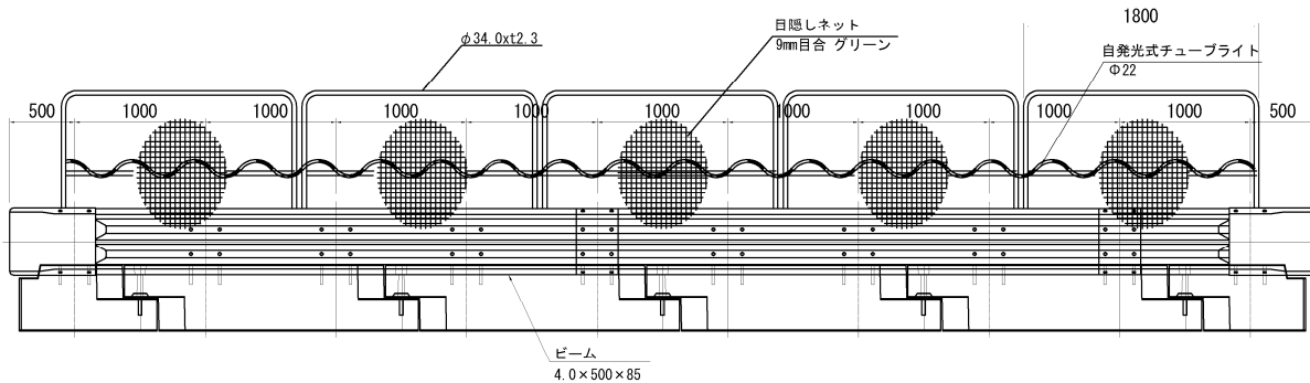
側面図
