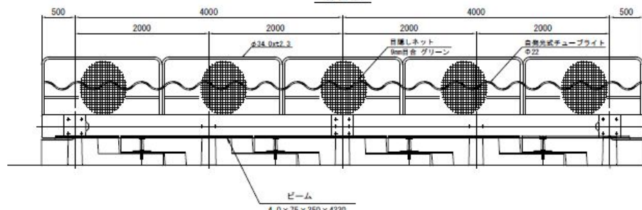
側面図
