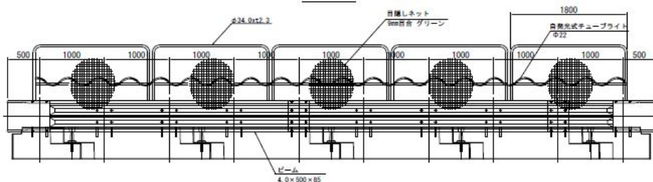
側面図
