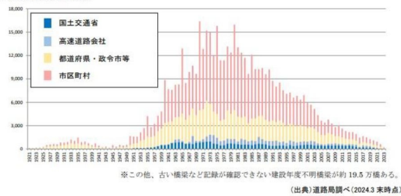
○ 建設後50年を経過した橋梁の割合
