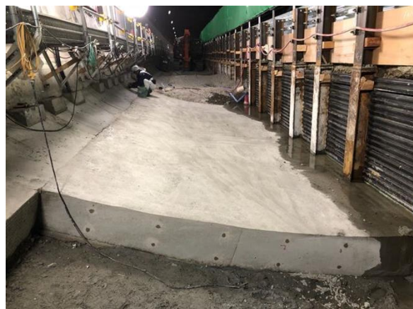
【長野道 一本松トンネルインバート設置工事状況】
