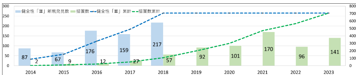
【省令点検2巡目の健全性「Ⅲ」発見数と措置数の推移】
