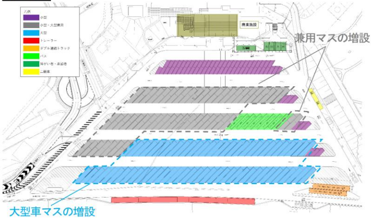
図-3 レイアウト変更状況 ( E4 東北道 那須高原 SA(下り) )
